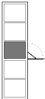
Klappe 380 / 450 mm
