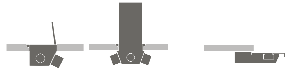
Steckerwanne einseitig und zweiseitig bedienbar Power outlet box with hinged lid, can be used from one or both sides
