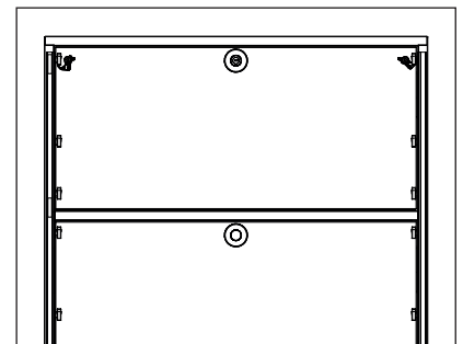
Einzelschliessung oder Zentralschliessung über alle Einbauten, Schlossposition frei wählbar.
