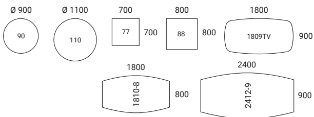
BESPRECHUNGSTISCH, Höhe 900 mm
